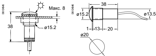
Фотоэлемент для щитового монтажа (15281) Крепится в вертикальном положении двумя винтами 2 Ø 4 мм снаружи щита
